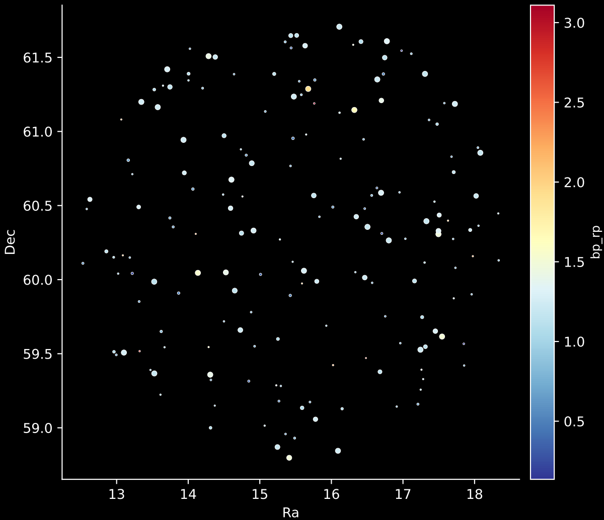
APOGEE DR17 Field: [CVZTILE_089+27_btx] Stars: 179
