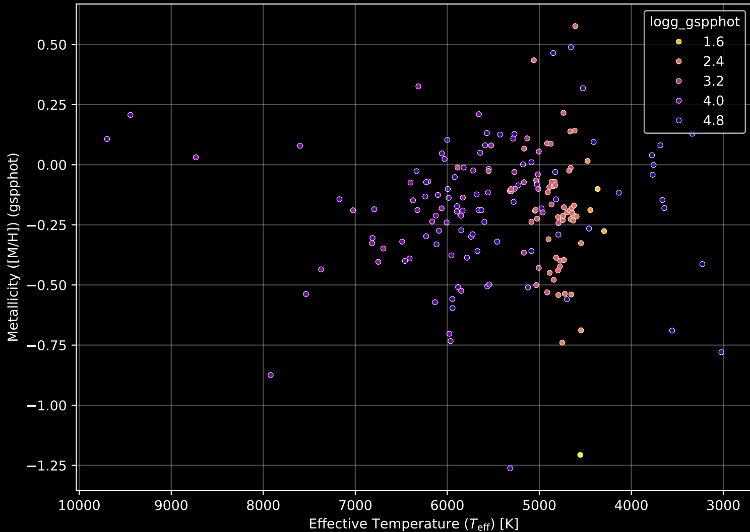
APOGEE DR17 Field: [CVZTILE_089+27_btx] Stellar Population Parameters (n= 179)
